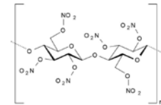
Struktur til nitrocellulose
